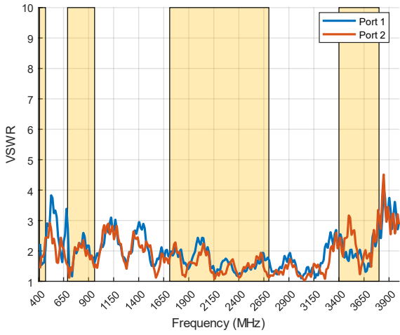
VSWR
